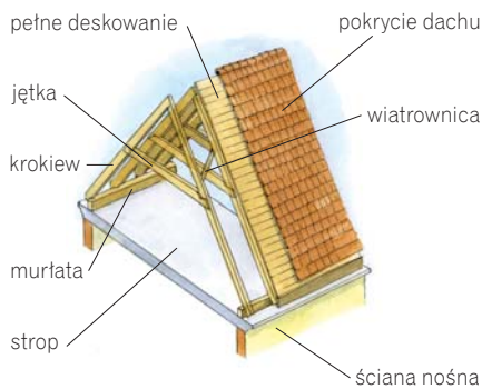
Dach o konstrukcji jętkowej
