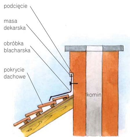
Obróbka blacharska komina
