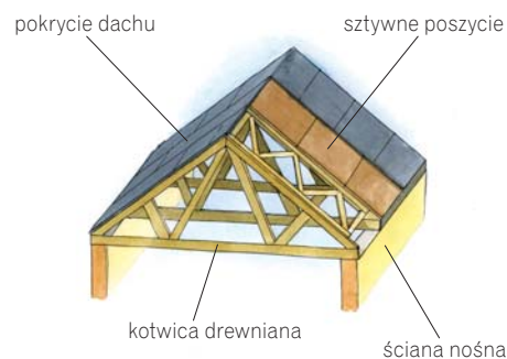
Konstrukcja dachu z deskowaniem z płyt
