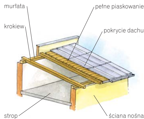
Konstrukcja dachu z deskowaniem po pokryciu dachowe
