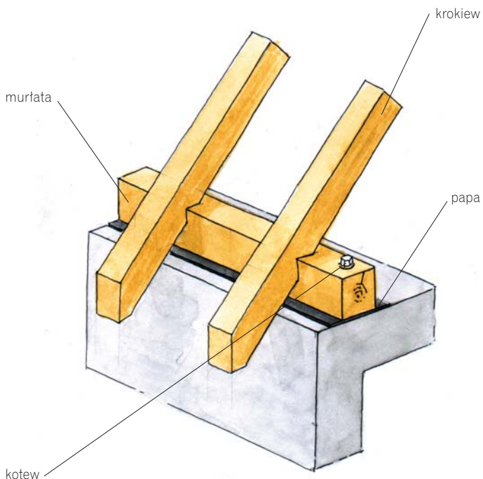
Sposób mocowania murłaty i oparcie krokwi na murłacie
