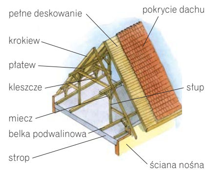
Dach o konstrukcji płatwiowo-kleszczowej
