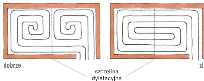
W rozplanowaniu obwodów grzewczych należy unikać skrzyżowań rur z dylatacją
