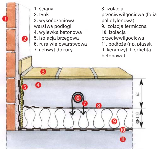
Układ warstw w podłodze z ogrzewaniem wodnym – podłoga na gruncie
