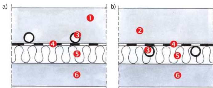
Układ warstw w podłodze z ogrzewaniem wodnym – podłoga na gruncie
