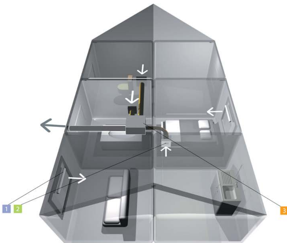
1 Nawiewniki powietrza 2 Kratki wyciągowe 3 Wentylator
