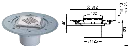
2 Nasadka do uszczelnień płynnymi masami izolacyjnymi z ABS, Rama □ 132 mm
