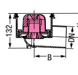
Ecoguss z syfonem, przepustowość 1,8 l/s, wysokość zamknięcia wodnego 50mm
