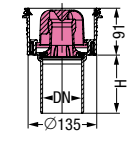
Practicus z PP, z syfonem, przepustowość 1,8 l/s, wysokość zamknięcia wodnego 50mm
