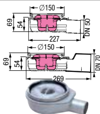
„Der Ultraflache” z ABS, odpływ boczny DN50/DN70, przepustowość 1,0 l/s, z syfonem, wysokość zamknięcia wodnego 30mm DN 50 45 700 DN 70 45 770
