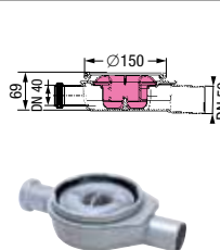
„Der Ultraflache” z ABS, odpływ boczny DN50, dopływ boczny DN40, przepustowość 1,0 l/s, z syfonem, wysokość zamknięcia wodnego 30mm 45 701
