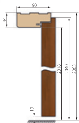
Ościeżnice blokowe
