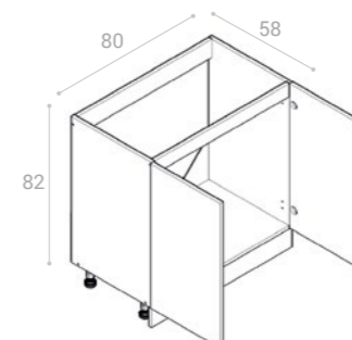
SZL/80
