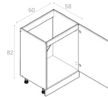
SZL/60
