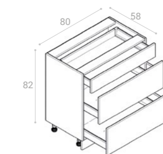
S/80/3 MODERNBOX
