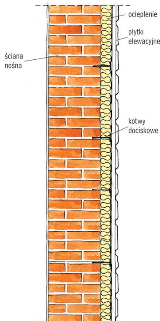
Płytki z piaskowca mogą być przyklejane do ocieplonej ściany tylko wtedy, gdy izolacja termiczna jest osłonięta siatką zbrojącą i dodatkowo przymocowana kołkami z talerzykami dociskającymi
