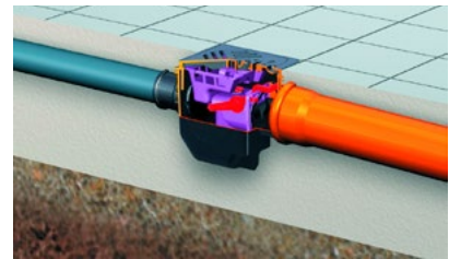
Zabudowa wpustu piwnicznego Drehfix z dwoma kłapami zwrotnymi
