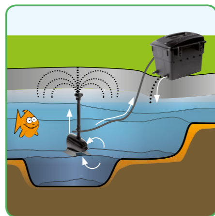
Rys. 1. Filtr AQUAEL pracujący na zewnątrz oczka
