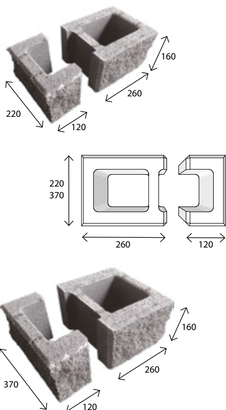
Bloczek słupkowy 370
