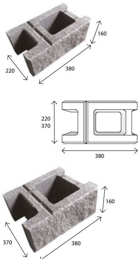
Bloczek cokołowy 370
