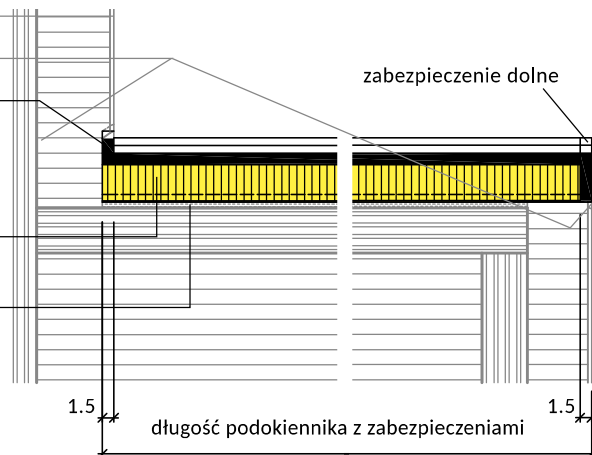
EJ z zabezpieczeniem górnym i dolnym Przekrój podłużny
