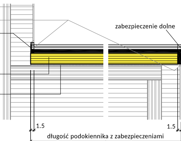
EL z zakończeniem górnym lub dolnym Przekrój podłużny
