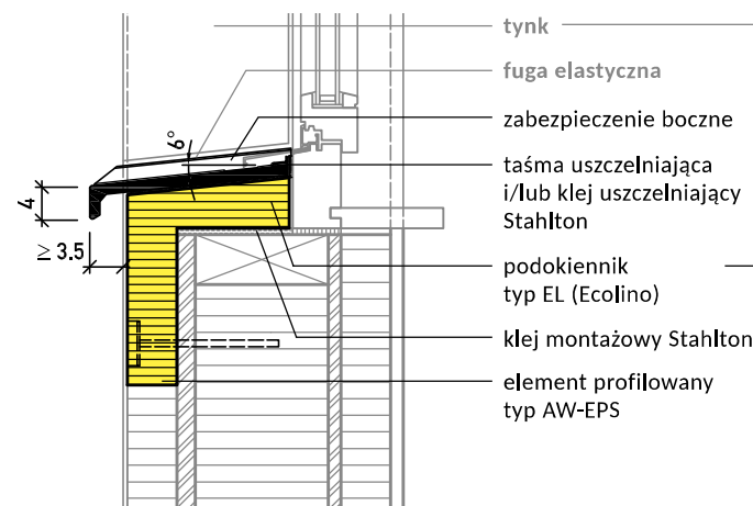
Podokiennik typ EL Przekrój pionowy
