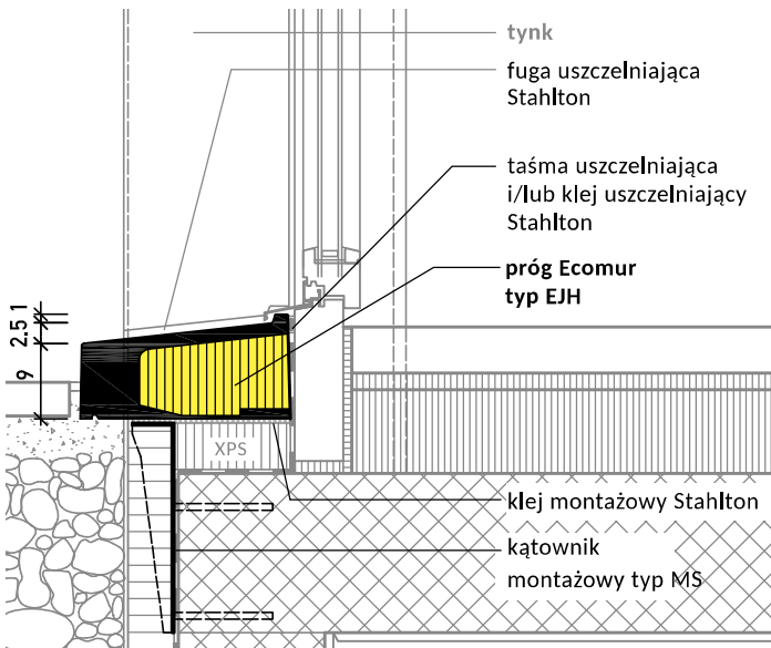
Próg typ EJH bez zakończenia bocznego Przekrój pionowy
