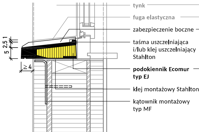
Podokiennik typ EJ z zabezpieczeniem bocznym Przekrój pionowy
