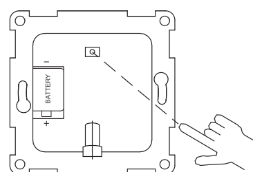
Czujnik IR
