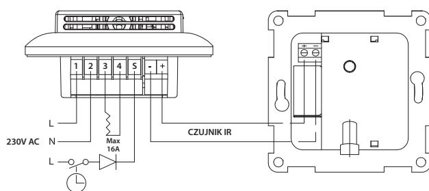
Schemat z trybem przeciwwamrożeniowym
