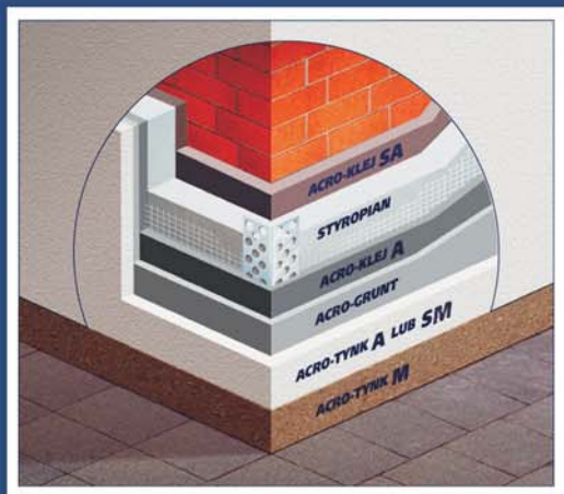
SCHEMAT SYSTEMU DOCIEPLEŃ
