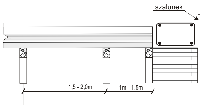
Rys 3. Podparcie montażowe bezpośrednio przy murze
