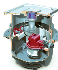
Przepompownia Aqualift F Unterflur
