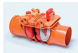
Zasuwa burzowa Staufix® z dwiema kłapami
