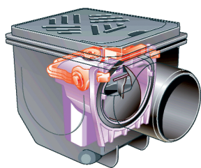
Wpust piwniczny Drehfix z dwiema kłapami zwrotnymi
