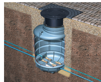
Studzienka wodomierzowa
