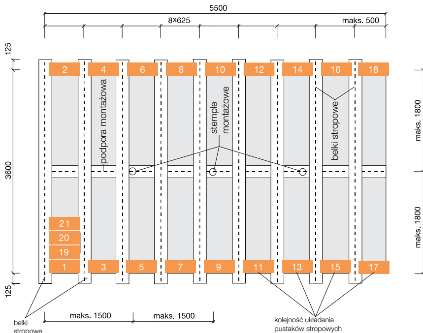
Schemat montażu stropu Porotherm 62.5 (przykład)
