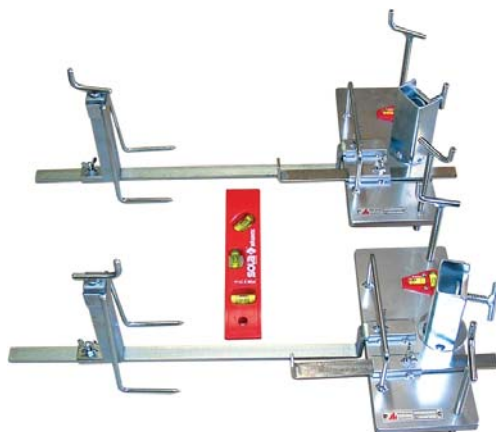
Stojaki do poziomowania pierwszej warstwy pustaków
