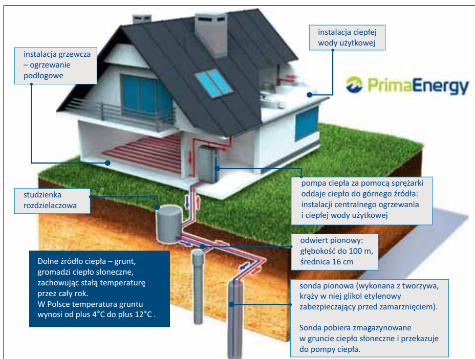
Schemat gruntuwej pompy ciepła PrimaEnergy
