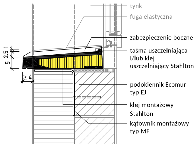
Typ EJ z zabezpieczeniem bocznym Przekrój pionowy
