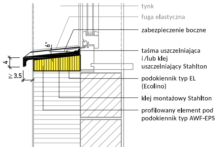
Typ EL (ECOLINO) Przekrój pionowy
