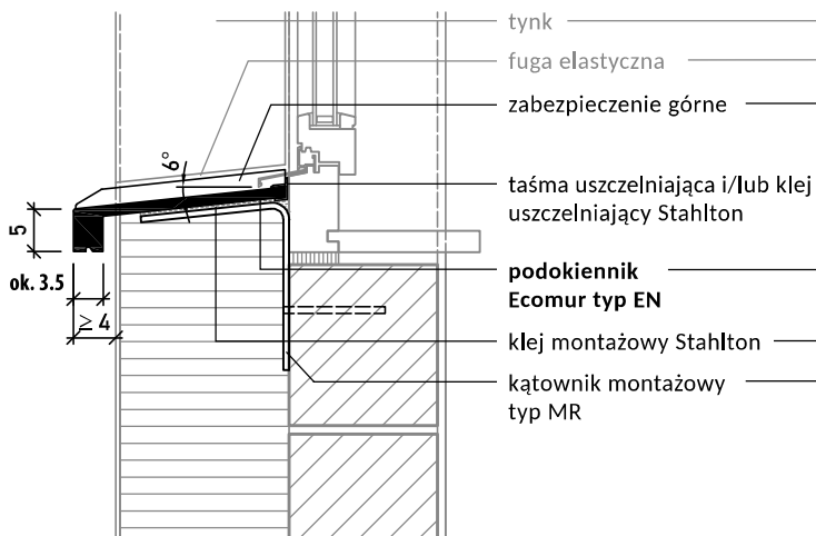
Typ EN z zakończeniem bocznym Przekrój pionowy
