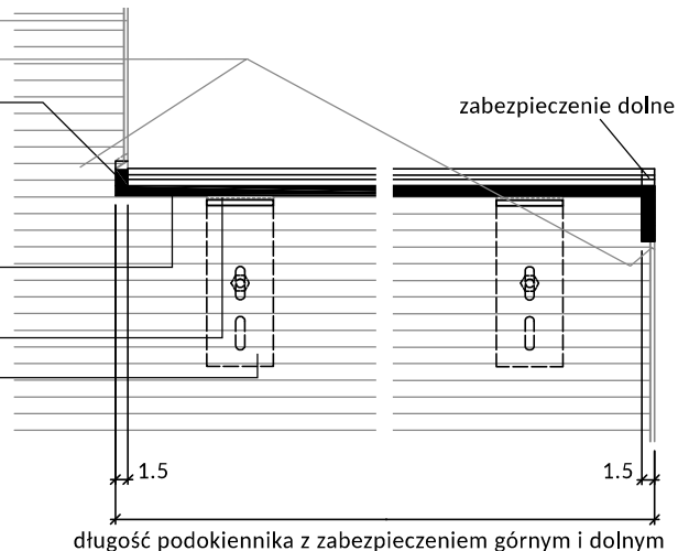
Z zabezpieczeniem górnym i dolnym Przekrój podłużny
