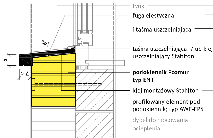
Typ ENT bez zabezpieczenia bocznego Przekrój pionowy
