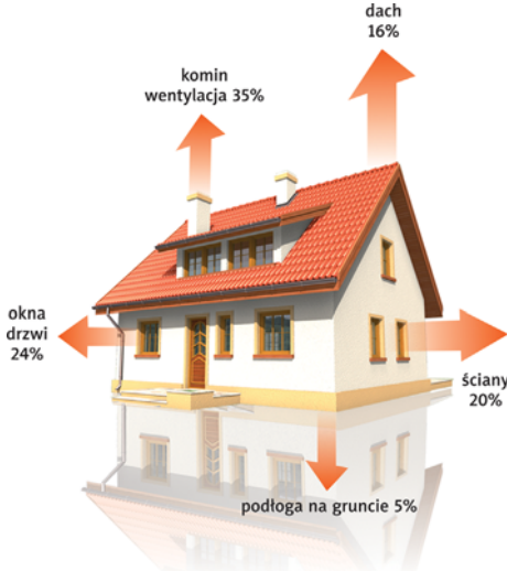
Rys. Schemat strat ciepła w budynku jednorodzinnym
