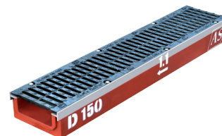
AS-A150T kl. C250 i D400 kN
