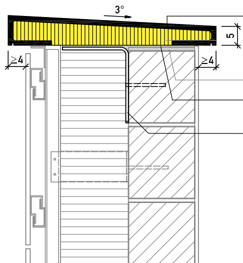
Czapa osłonowa typ EBJ z wkładką termiczną z EPS Przekrój pionowy
