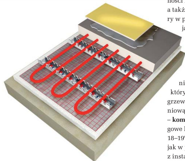
Ogrzewanie podłogowe
