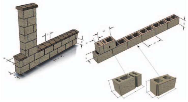
Prześło ze słupkiem 39 x 19
