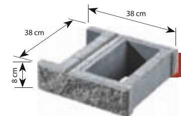
Pustak łupany (podmurówkowy) symbol: G1 waga: ok. 13 kg
