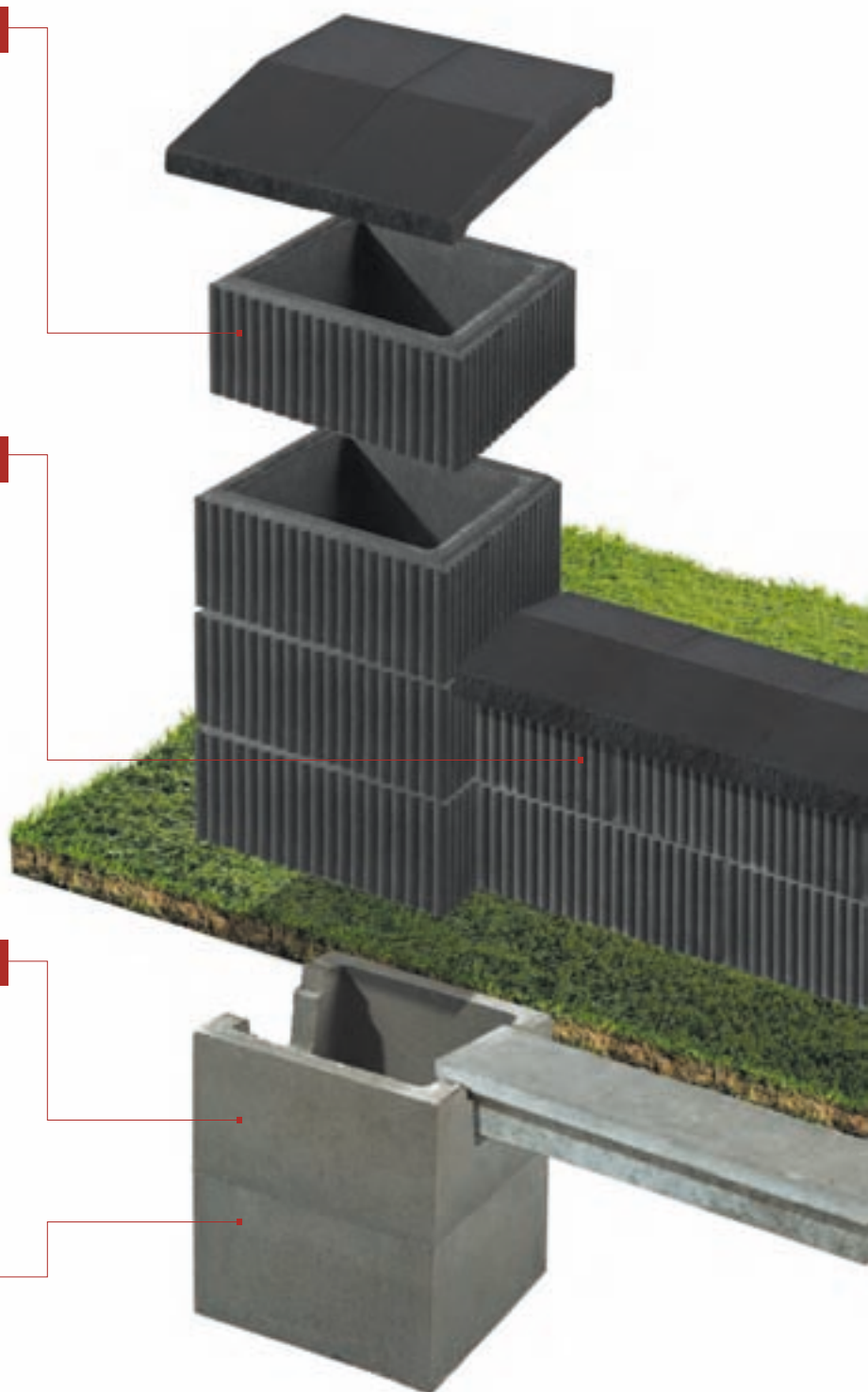
Pustak fundamentowy (z wpustem) symbol: D2 waga: ok. 30 kg
