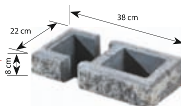
Pustak łupany (słupkowy) symbol: F2 waga: ok. 8 kg
