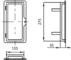
drzwi wyczystki
