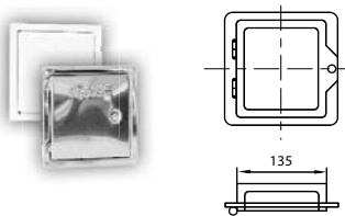
drzwi wyczystki
