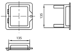
drzwi wyczystki
