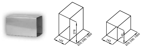
przedłużenie wyczystki
