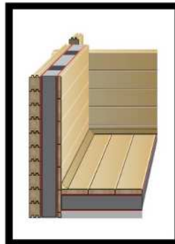
Izolacja od wewnątrz
