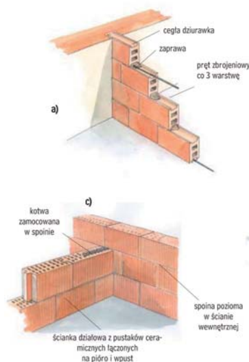
Połączenie ceramicznych ścian działowych z nośnymi: a – w bruzdzie wykonanej w ścianie nośnej, b – za pośrednictwem tzw. strzępi, c – metalowymi kotwami, wkręcanymi lub wmurowanymi w ścianę nośną
