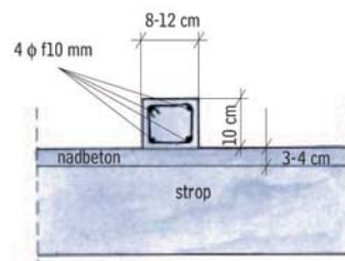
Żelbetowe żebro na gotowym stropie – wzmocnienie pod ściankę działową
