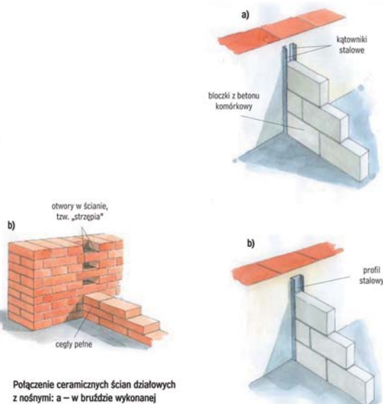
Połączenie ścian działowych z betonem komórkowym z nośnymi: a – za pomocą kątowników metalowych, b – za pomocą profili o przekroju U
