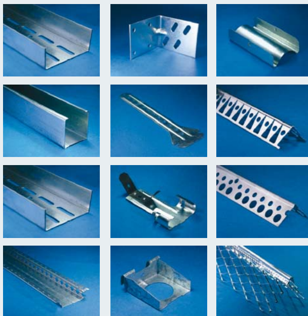
Kompletny system akcesoriów do systemów suchej zabudowy składa się z wielu elementów
