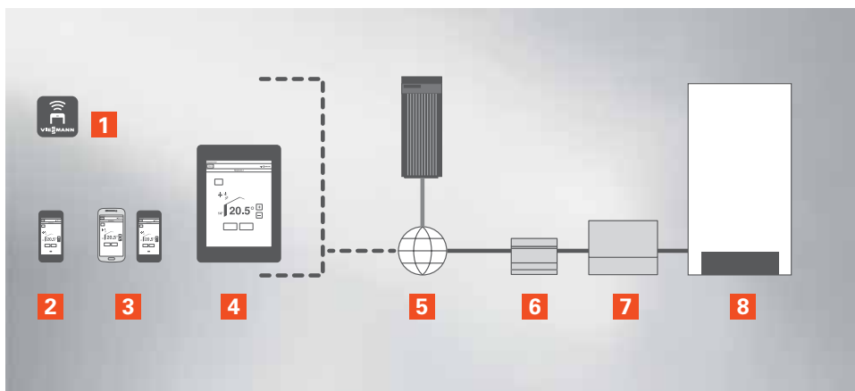
Schemat instalacji modułu Vitocom 100 LAN
