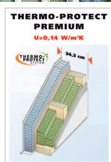
„PASYWNE” ŚCIANY
